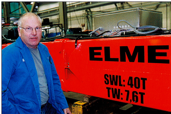
Ett containerlyftok är en kvalificerad teknisk produkt utsatt för extrem utmattningsbelastning. Oken ska ha så låg vikt som möjligt och samtidigt tåla så stor belastning som möjligt. – Det kan se rätt enkelt ut, men kraven är mycket stora, säger produktionsledaren Per Eric Larsson på ELME.
